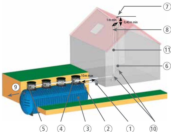
Schéma de raccordement de la ventilation haute pour une micro-station ACTIBLOC® 16EH (14000 DP).
