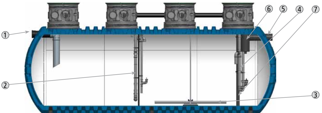
Vue de coupe d'une micro-station ACTIBLOC® 16EH (14000 DP).
